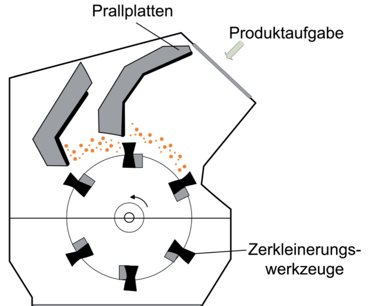
Abbildung 5: Schema einer Prallmühle: Das Mahlgut wird zwischen den feststehenden Prallplatten und den Schlagleisten des sich drehenden Rotors zerkleinert.
