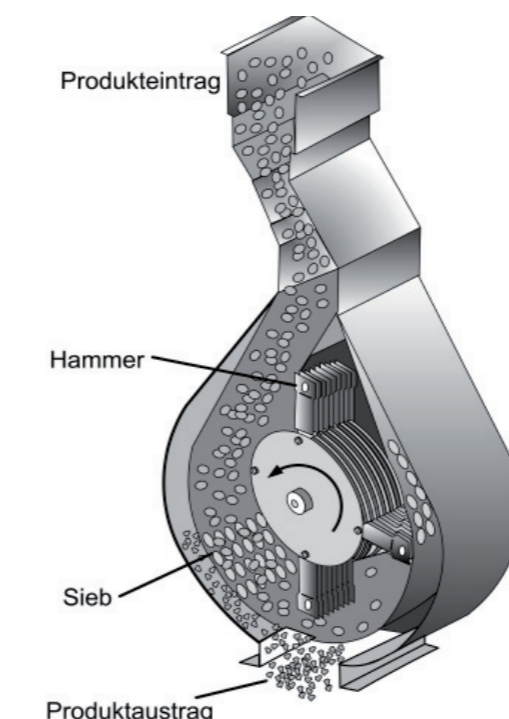
Abbildung 2: Schematische Zeichnung einer Hammermühle
