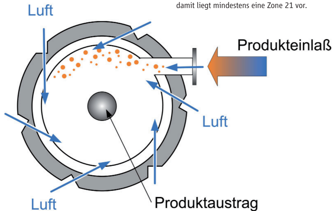
Abbildung 10: Prinzip einer Luftstrahlmühle
