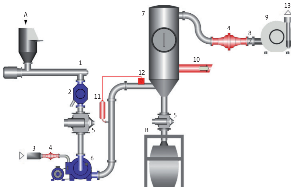
Abbildung 7: Anlagenbeispiel für eine schnelllaufende Mühle ausgelegt für einen reduzierten Explosionsüberdruck durch Explosionsdruckentlastung in Kombination mit explosionstechnischer Entkopplung.
