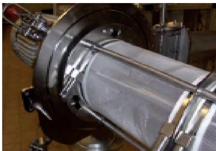
Abbildung 24: Prinzip einer Wirbelstromsiebmaschine (oben) Das linke Bild zeigt den Siebkorb. [Bild: AZO® GmbH & CO KG]
