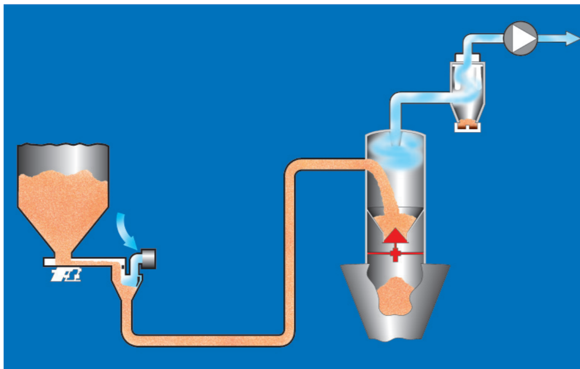
Abbildung 20: Anwendungsbeispiel eines Schwerekraftabscheiders als Primärabscheider in der pneumatischen Förderung [Bild: AZO® GmbH & CO KG]
